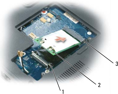
1 Ganchos de fijación 2 Conectores de antena (2) 3 Conector de minitarjeta
